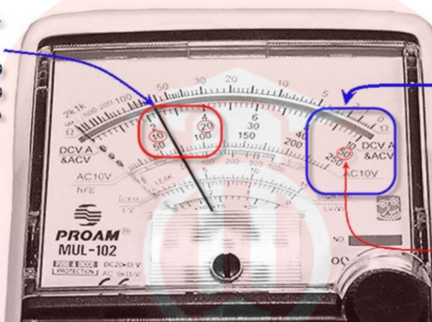
شکل ۱۳ - نحوه خواندن ولتاژ از مولتی متر آنالوگ ۱
