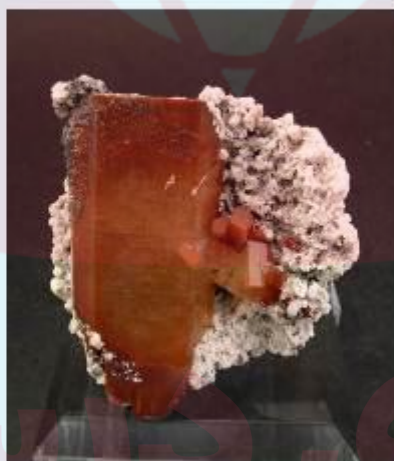
توپاز
