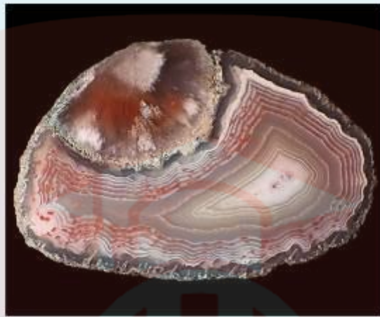
کلسدونی
