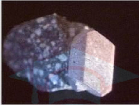
ارتو کلاز
