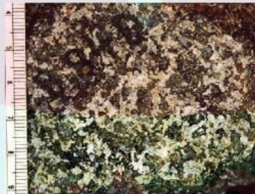
گابرو
