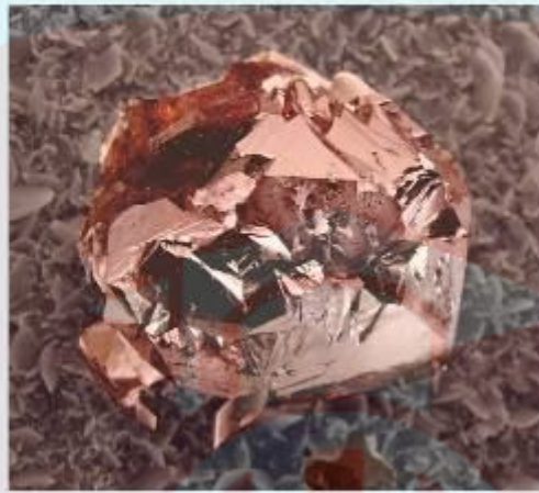
اسفالریت
