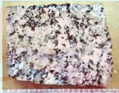
گرانیت
