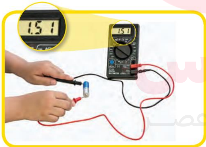
شکل ۶- اندازه گیری اختلاف پتانسیل دو سر باتری
